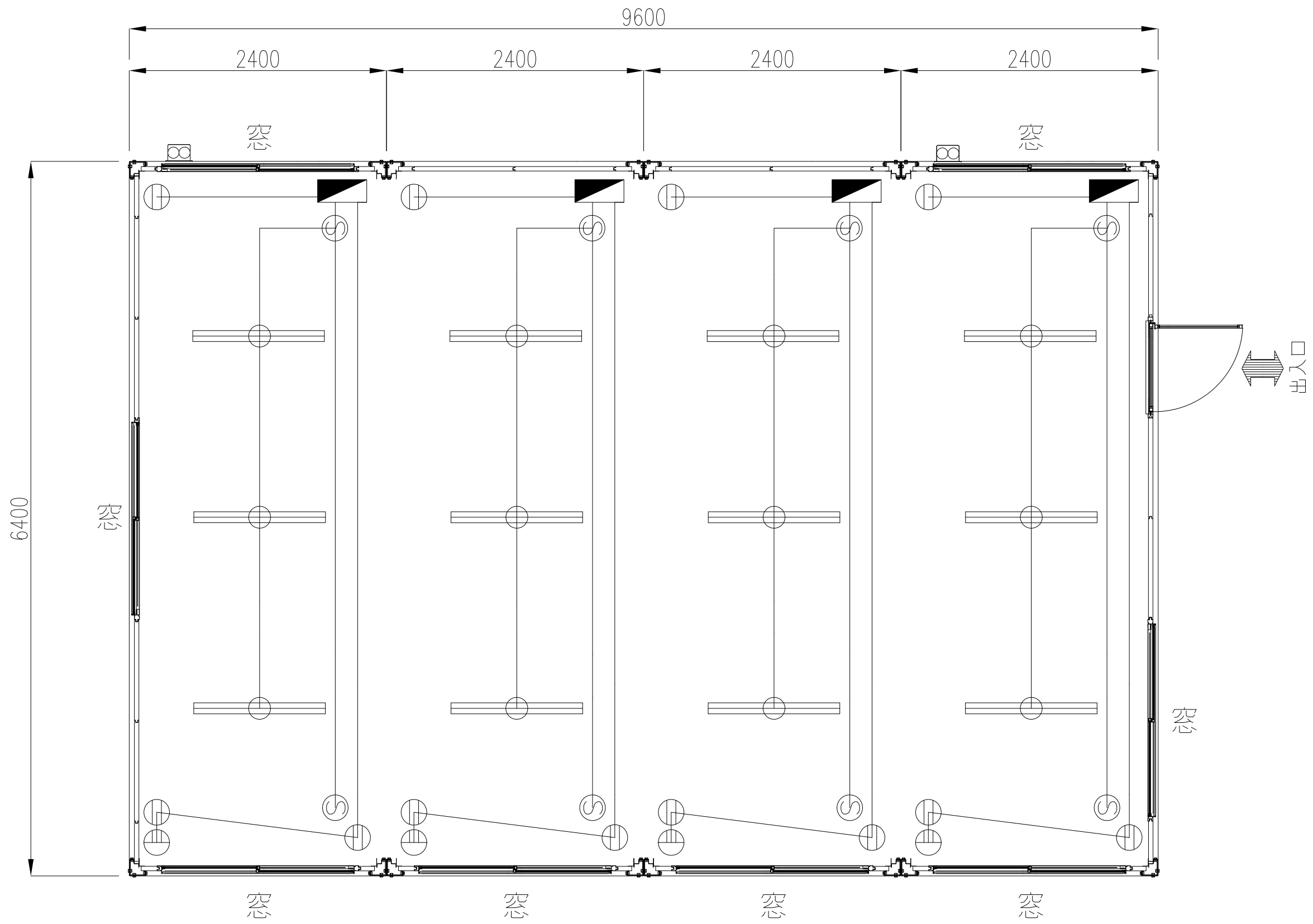
No588 (端棟)
