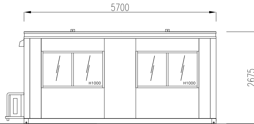
左側面図
