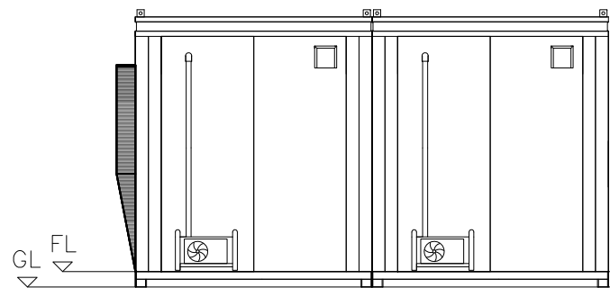
背面図
