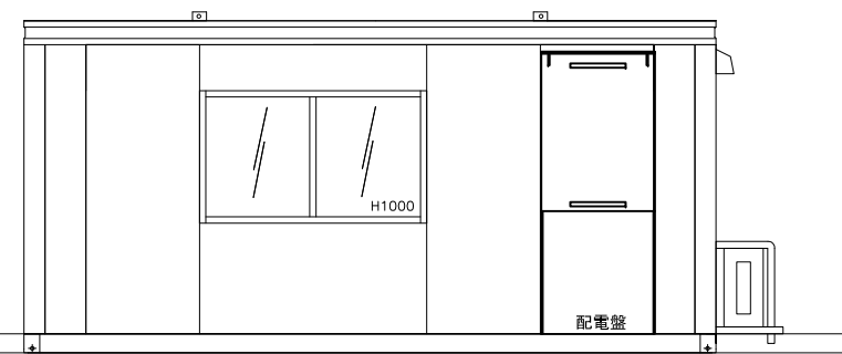
右側面図
